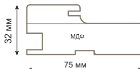
Коробка ТехноМДФ 35 (75*32) Frame TehnoMDF 35 (75*32)
