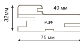
Наличник Телескоп Trim Telescope
