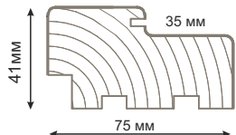
Коробка Классика 35(41*75) Frame Classics 35(41*75)
