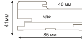
Коробка Телескоп 40(41*85) Frame Telescope 40(41*85)
