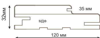
Коробка Телескоп 120 Frame Telescope 120
